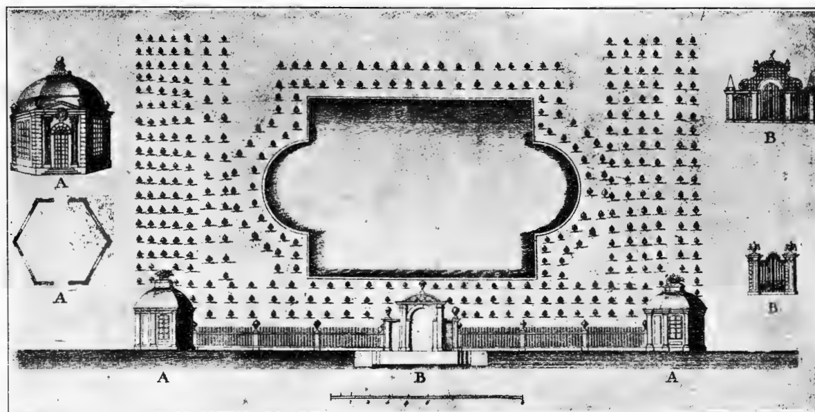
Проектъ сада архитектора Трезини.
