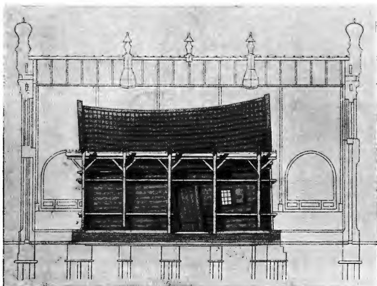
Разрѣзъ каменнаго строенія и домина Петра I. Въ современномъ видѣ.
