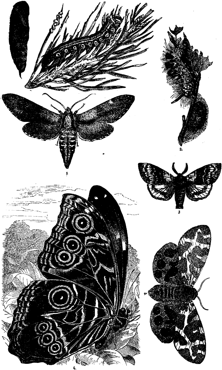
1. Сосновый бражник ( Sphinx pinastri ) съ яичками, гусеницей и куколкой. 2. Колонъ и гусеница буюого шелкопряда. 3. Буюог шелкопряда ( Dasychira rudibunda ), самецъ. Ест. вел. 4. Неоптолемъ ( Morpho Neoptolemus ). Ест. вел. 5. Буюог медвѣдь ( Arotia Caja ).
