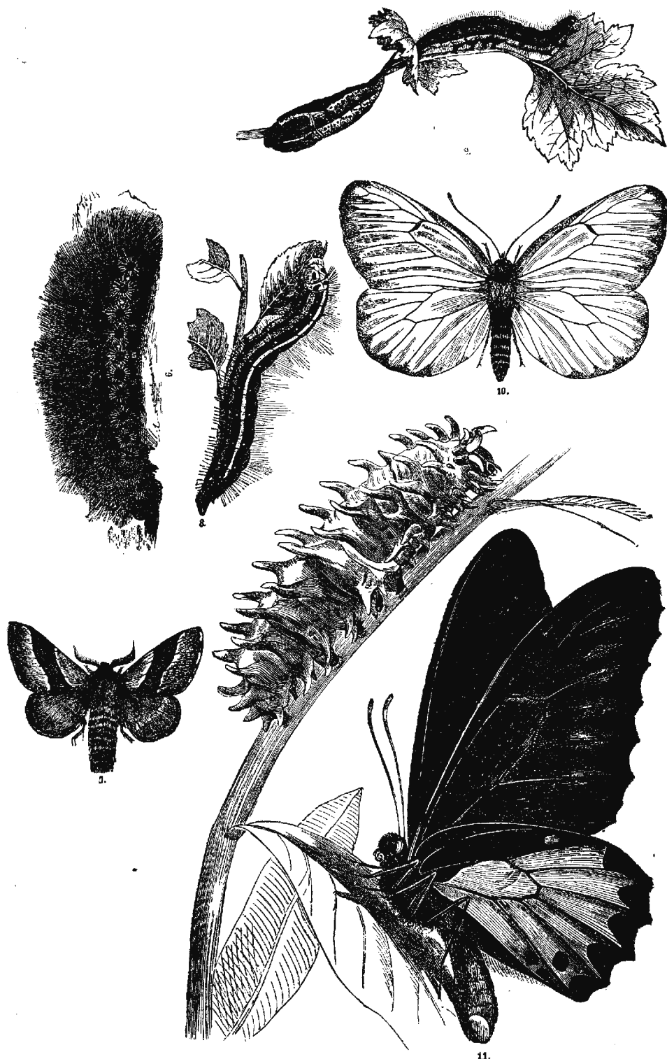
6. Гусеница бурога медвѣда ( Arotia saja ). Ест. вел. 7. Кольчатый шелкопрядъ ( Lasiocampa neustria ), самецъ. Ест. вел. 8. Гусеница кольчатого шелкопряда. 9. Куколка и гусеница боярышницы. 10. Боярышница ( Pieris crataegi ). Ест. вел. 11. Ornithoptera Amphrisus съ гусеницей. Ест. вел.
