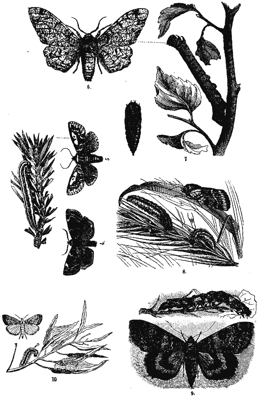
4. Иллимовая совка ( Cosmia diffracta ). Ест. вел. 5. Сосновая свиноголовка ( Trachea piperperda ) с гусеницей. Ест. вел. 6. Березовая пяденица ( Agryphidasya betularia ). Ест. вел. 7. Куколка и гусеница березовой пяденицы. 8. Пырейная свиноголовка ( Madena basilinea ) с гусеницами. Ест. вел. 9. Красная орденская совка ( Catocala picta ) с гусеницей, \frac{2}{3} ест. вел. 10. Рапсовая огневка ( Botys margaritalis ) с гусеницей. \frac{2}{3} ест. вел.
