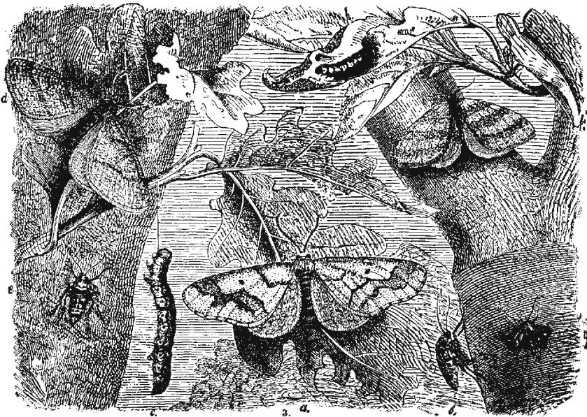
1. Сосновая пяденица ( Fidonia piniaria ) съ гусеницей. Ест. вел. 2. Лиственничная моль ( Coleophora laricella ), увел., и верхушечный побѣг лиственницы съ выѣденными хвоеми. 3. Большая дубовая пяденица ( Hibernia defoliaria ): a —самецъ, b —самка, c —гусеница. Hibernia aurantiaria : d —самецъ, e —самка. Малая дубовая пяденица ( Larentia brumata ): f —самецъ, g —самка, h —гусеница. Ест. вел.
