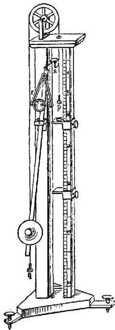
Атвудова машина.
