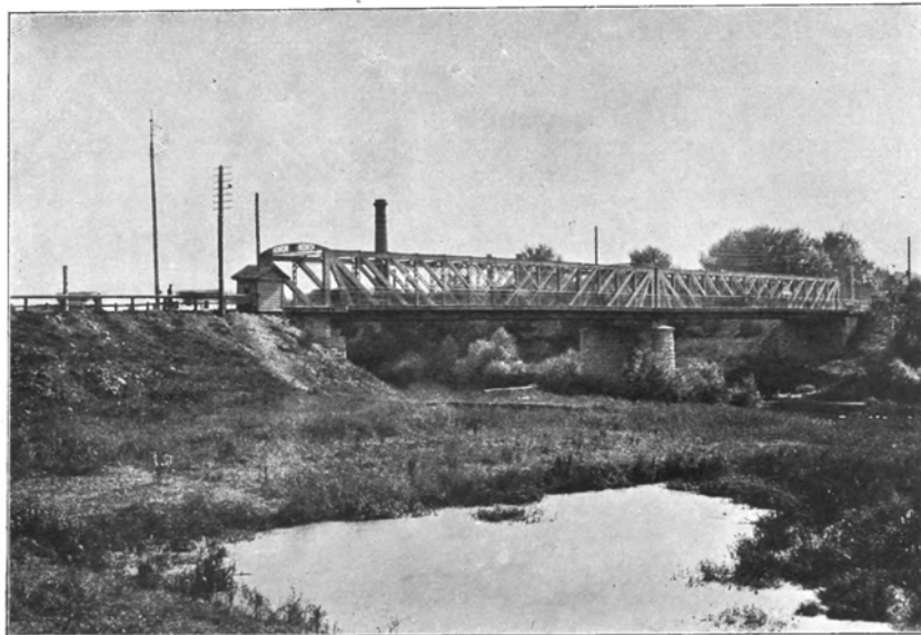
Гор. Тула. Железнодорожный мостъ черезъ р. Упу, построенный губернскимъ земствомъ.
