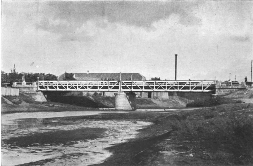
Мелитопольское уездное земство, Таврической губ. Железный мостъ черезъ рѣку Молочную, въ гор. Мелитополь. Построенъ въ 1890 году.
