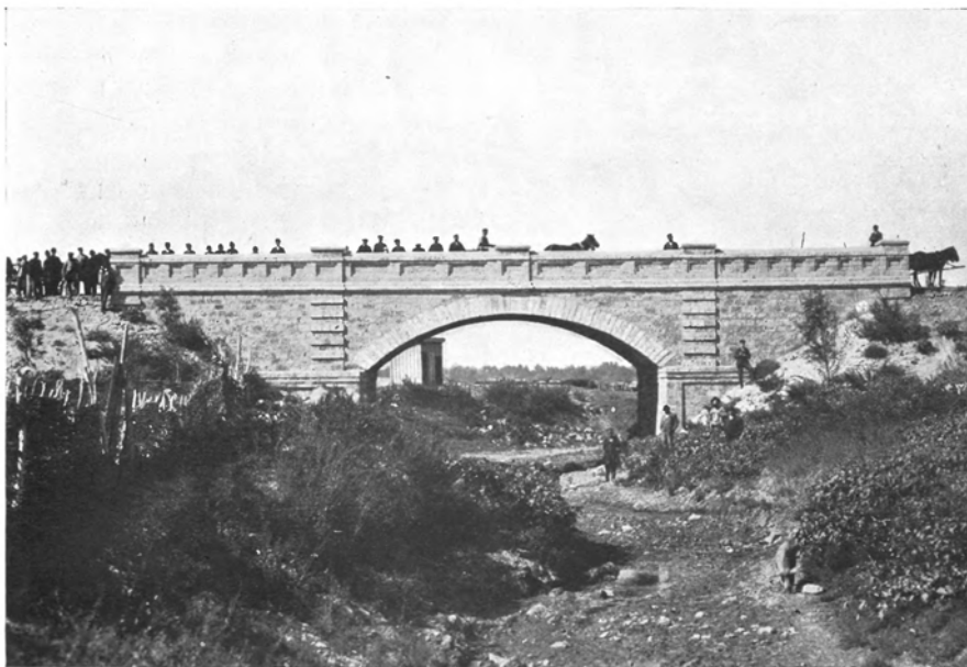
Мелитопольское уездное земство, Таврической губ. Каменный арочный мостъ черезъ балку, впадающую въ р. Днѣпръ, въ селѣ Большой Лепатихѣ. Построенъ въ 1900 г.
